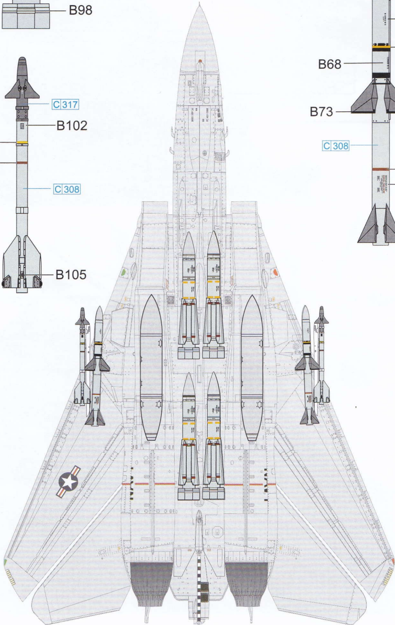
AIM-9
